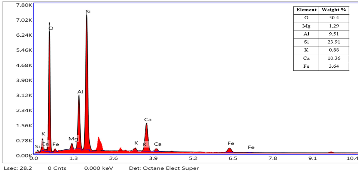
Şekil 7. Kil numunesin SEM-EDX elementel Analizi
