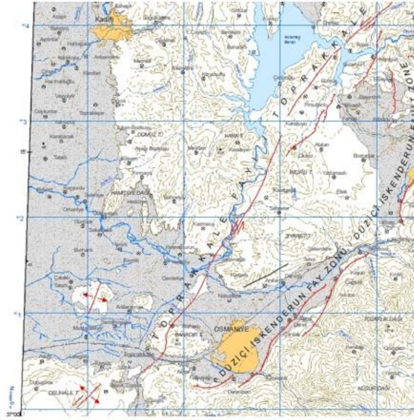
Şekil 10. Sol yönlü doğrultu atımlı Toprakkale fayının ve daha doğudaki İskenderun-Düziçi Fay hattının uzanımını gösterir eşyükselti haritası (MTA harita arşivinden).
