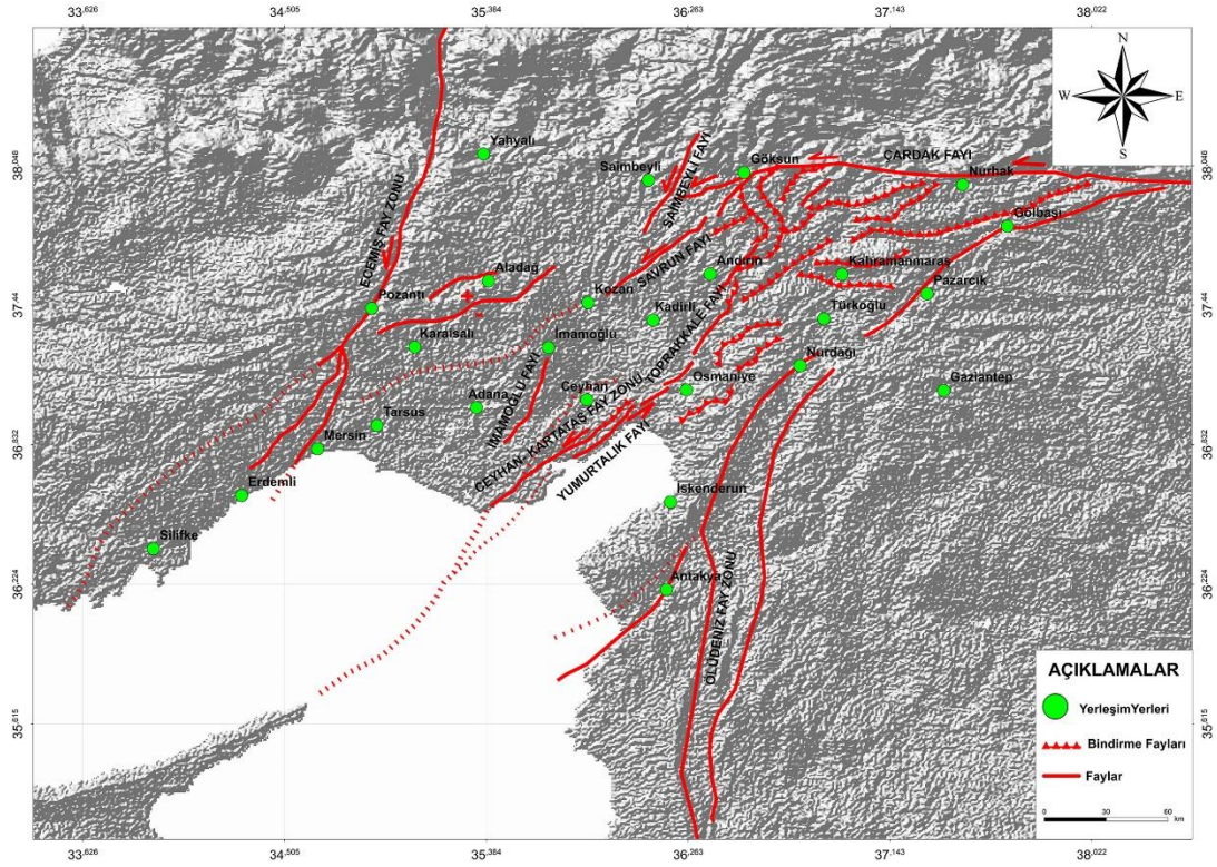
Şekil 6. İnceleme bölgesindeki aktif fayların geometrileri (Ünlügenç ve diğ., 2023).
