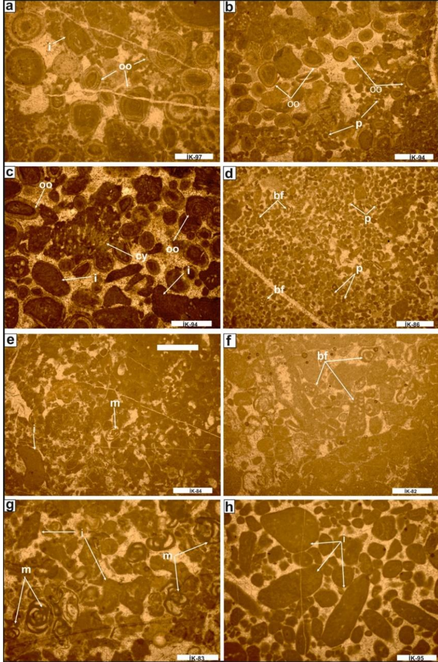
Şekil 9. Akseki Formasyonu'nun mikrofasiyes toplulukları. a-c) Oolitik istiftaşı/tanetaşı (MFT-4), oo:oolit; i:intraklast, p:peloid, cy:Cayeuxia (alg); d) Pelloidal istiftaşı/tanetaşı
